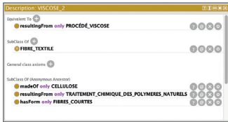
(d) dimension conceptuelle - Fragment d'ontologie en OWL
